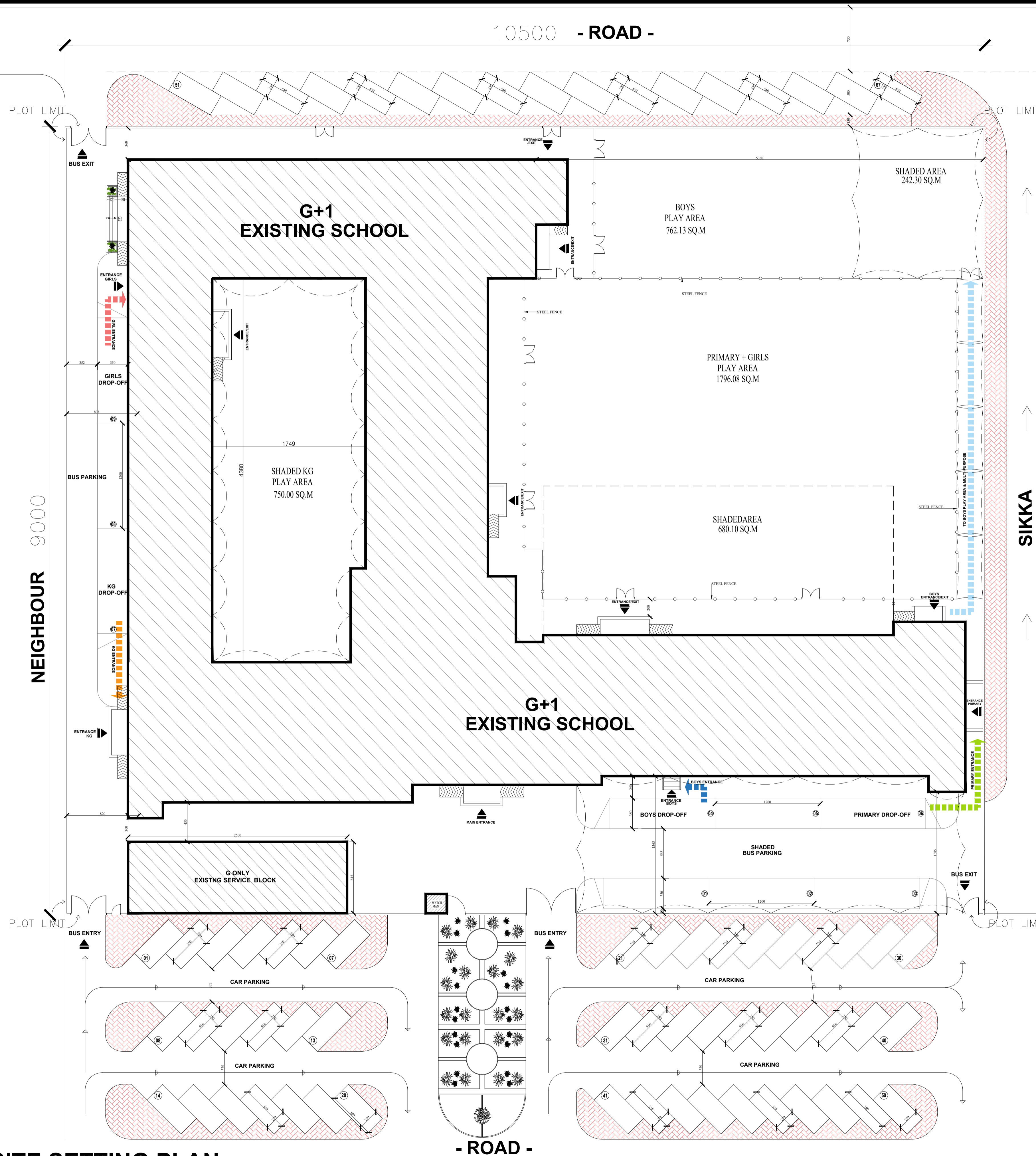
1 SITE SETTING PLAN A-100 SCALE N.T.S
